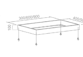
socos/zócalos
