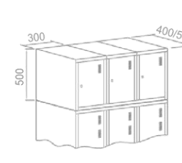
sobrepostos/altillos
